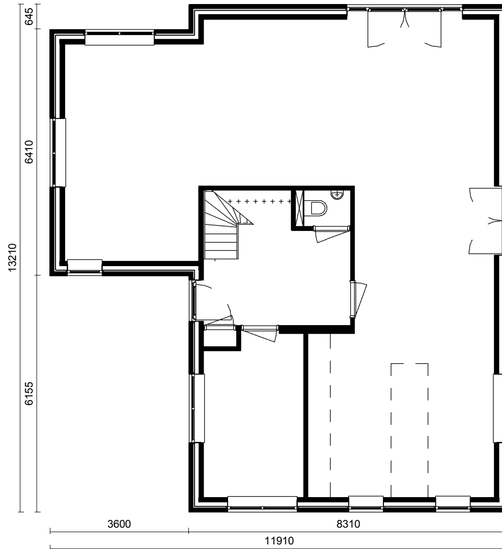
Begane grond
