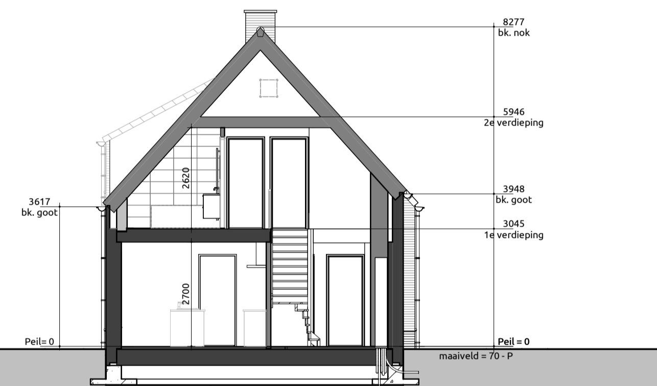
Doorsnede B-B
