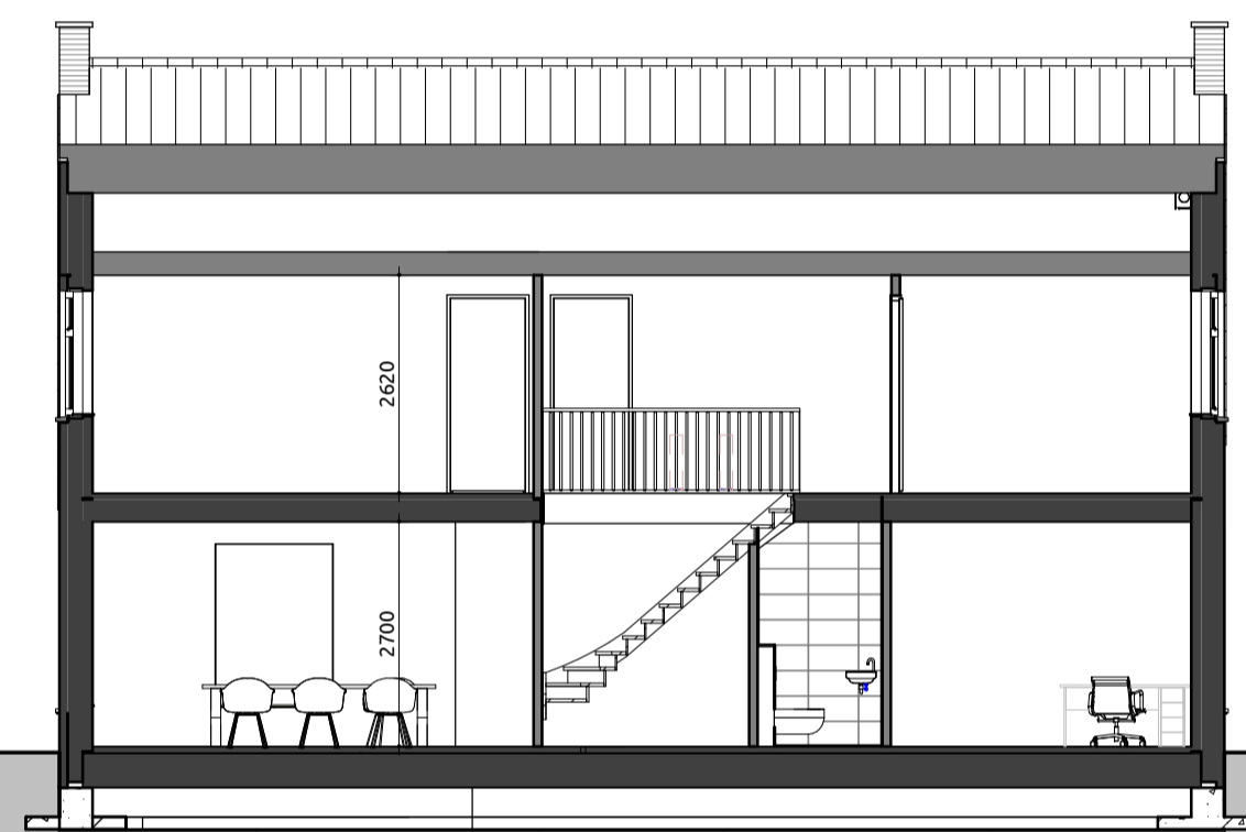
Doorsnede A-A
