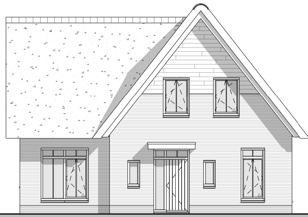
Voorgevel
