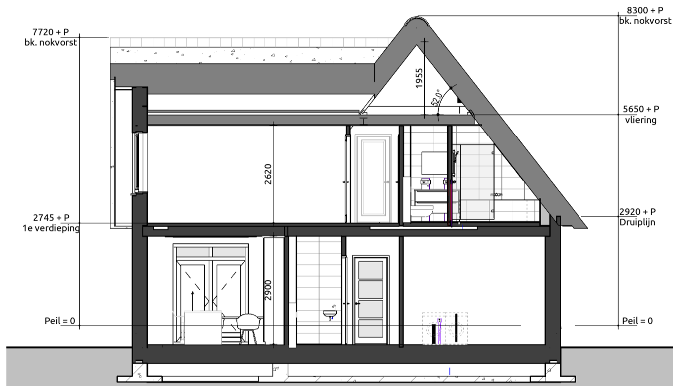
Doorsnede A-A
