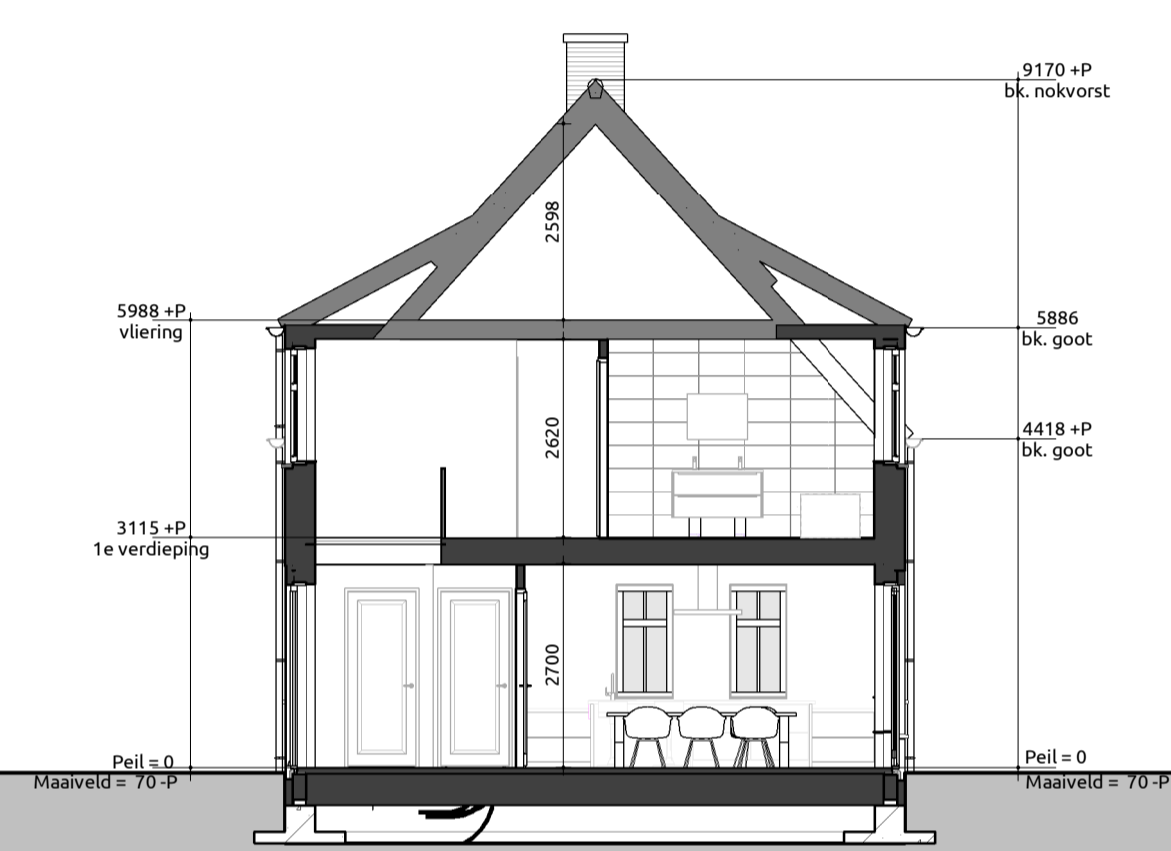
Doorsnede B-B
