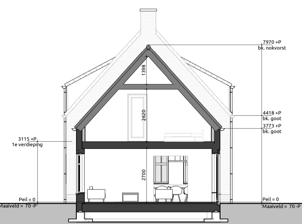
Doorsnede C-C
