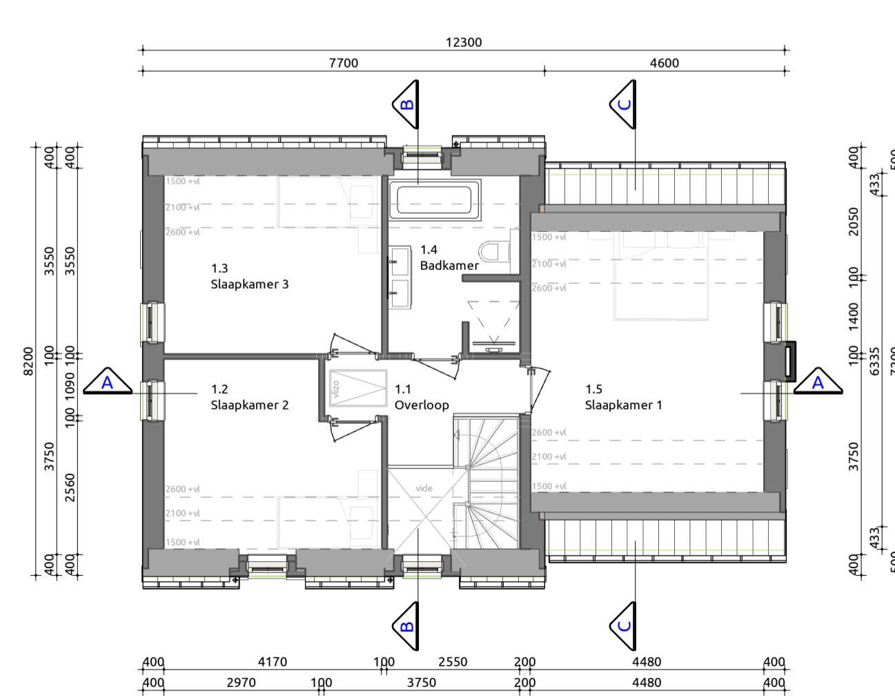
Eerste verdieping
