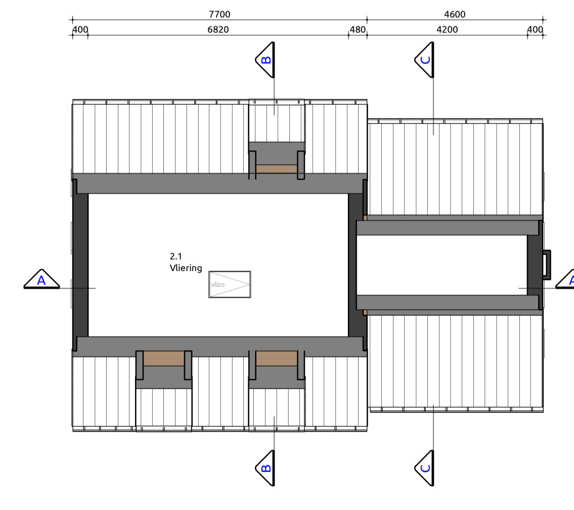
Tweede verdieping
