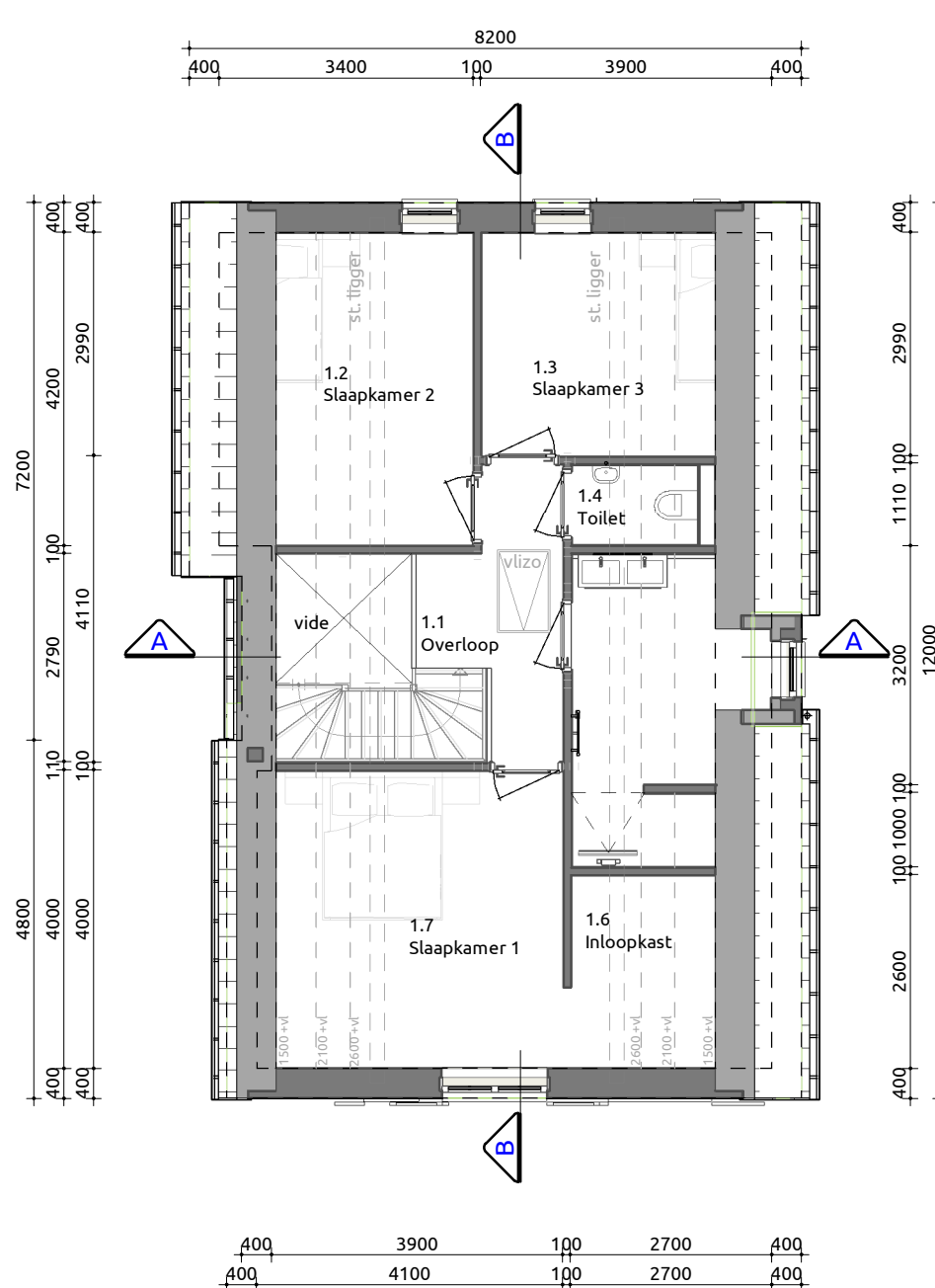
Eerste verdieping
