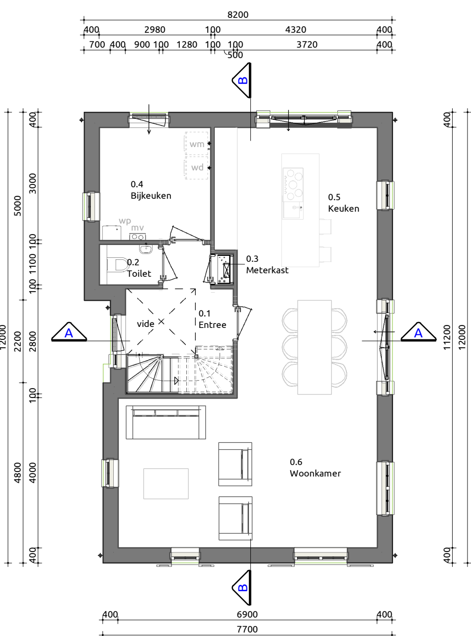
Begane grond
