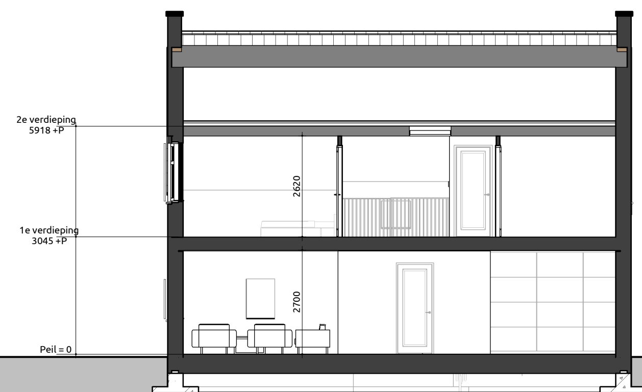
Doorsnede B-B
