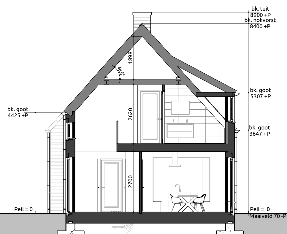
Doorsnede A-A
