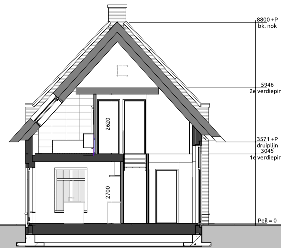
Doorsnede B-B
