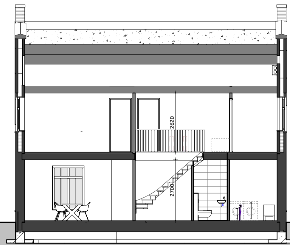
Doorsnede A-A
