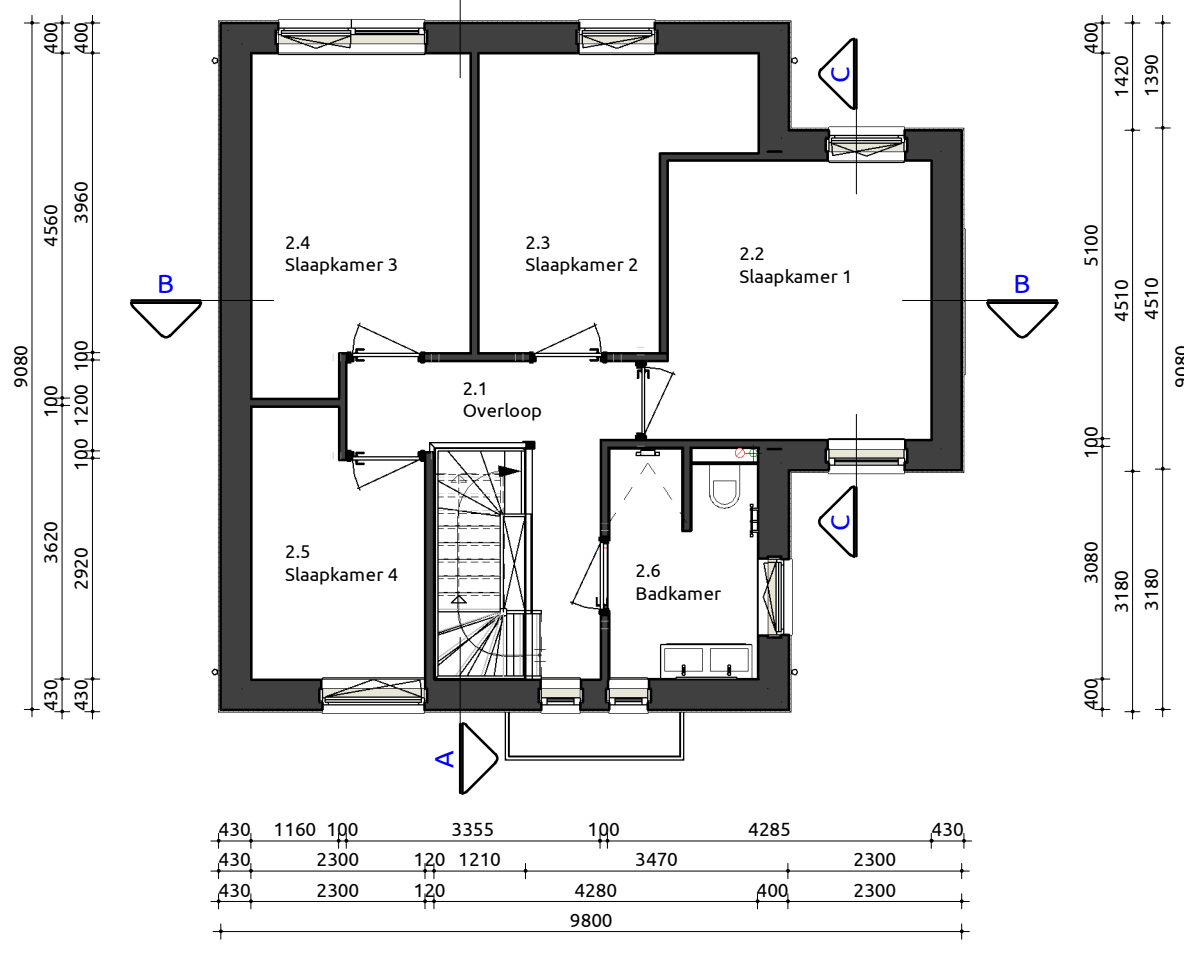
Eerste verdieping 1:100
