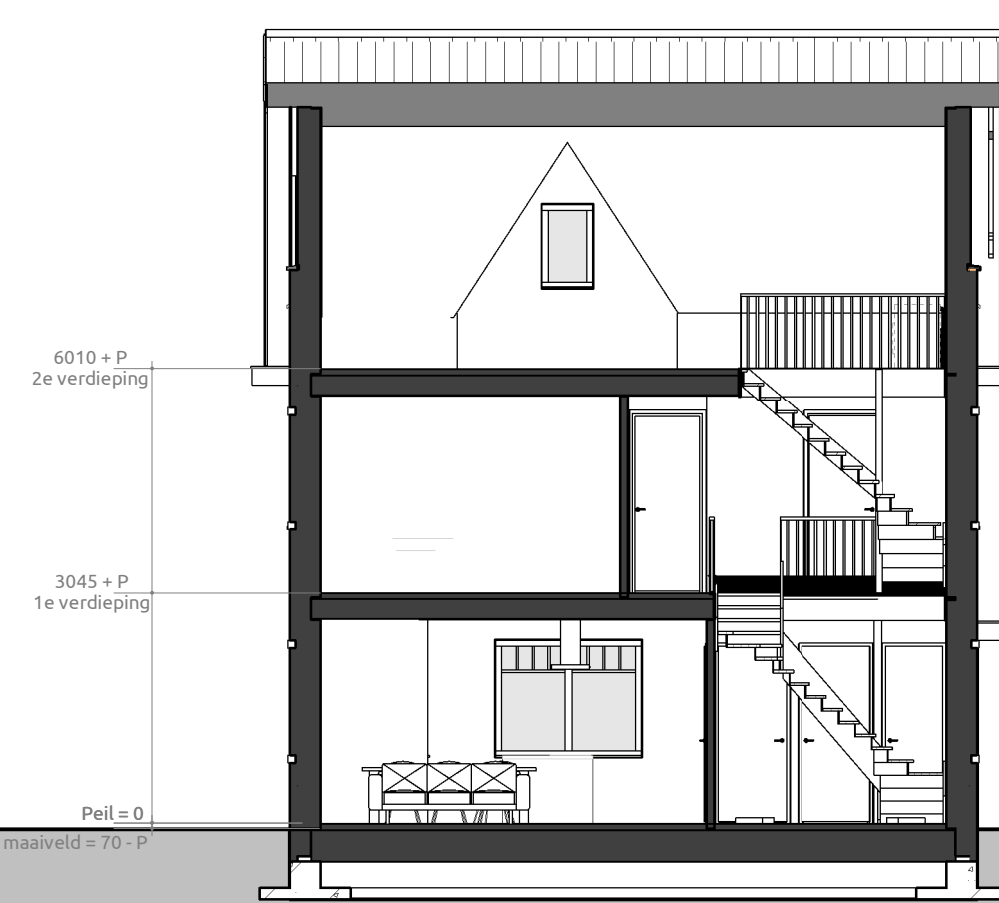
Doorsnede A-A 1:100
