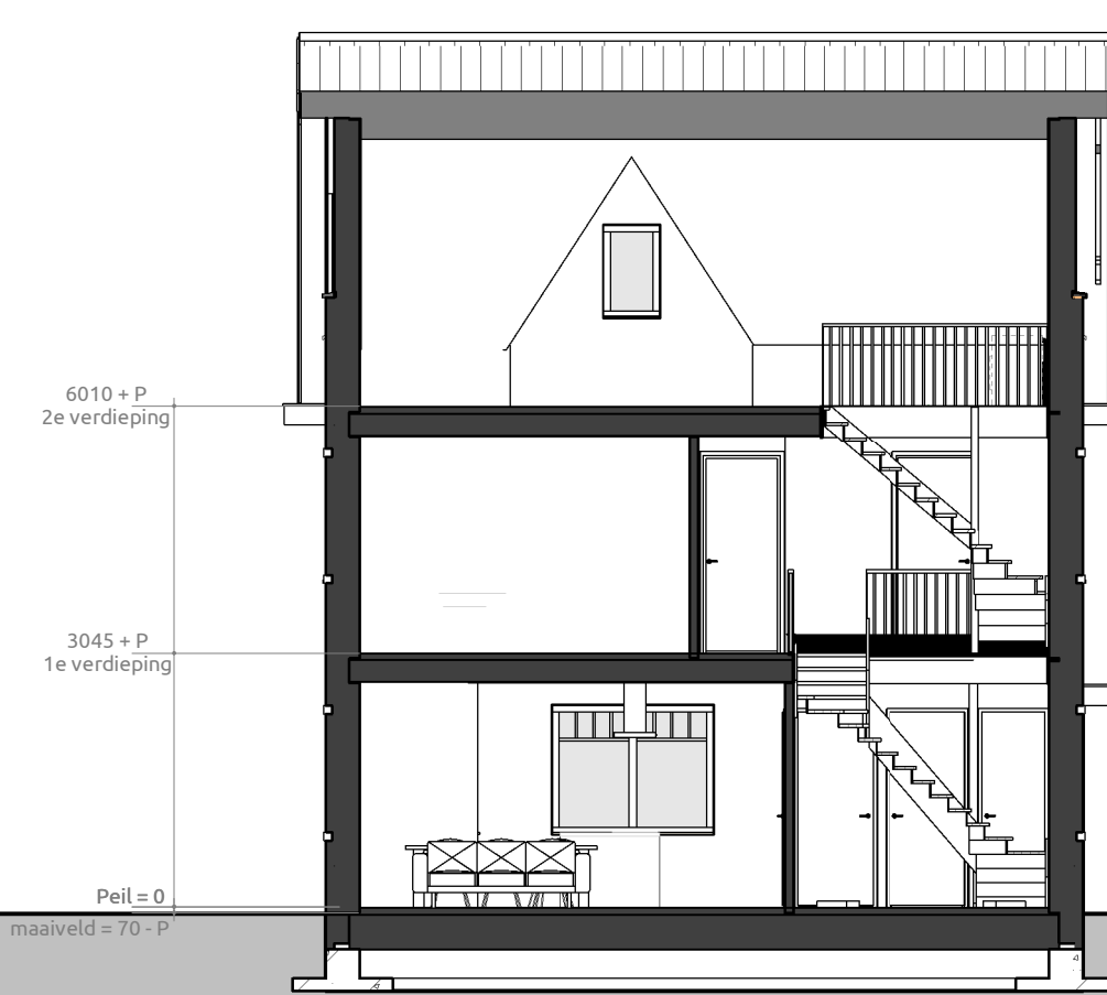
Doorsnede A-A 1:100
