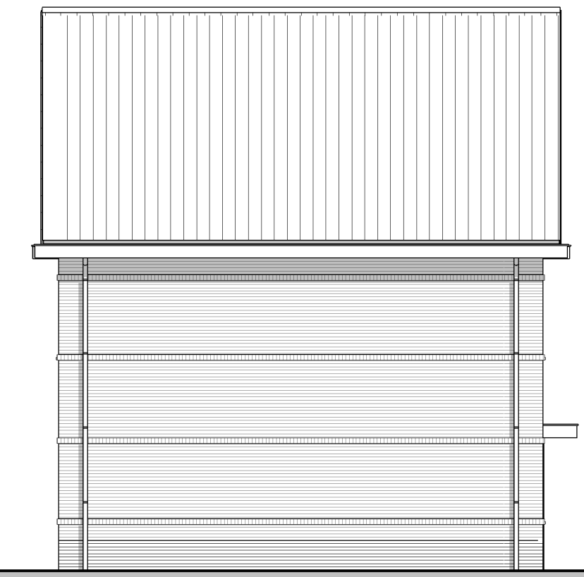
Linkergevel 1:100
