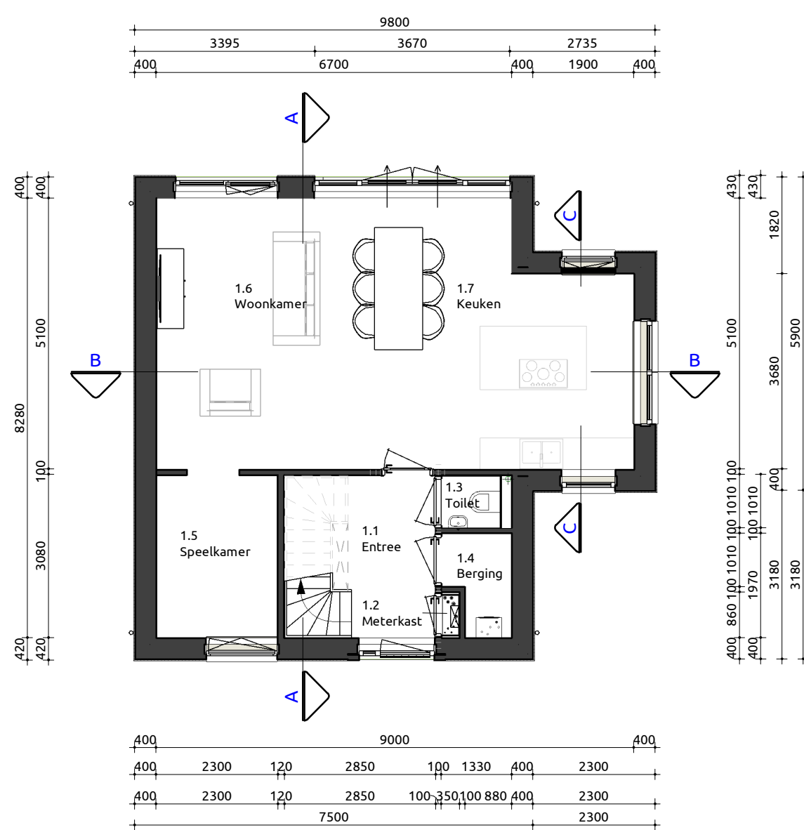
Begane grond 1:100
