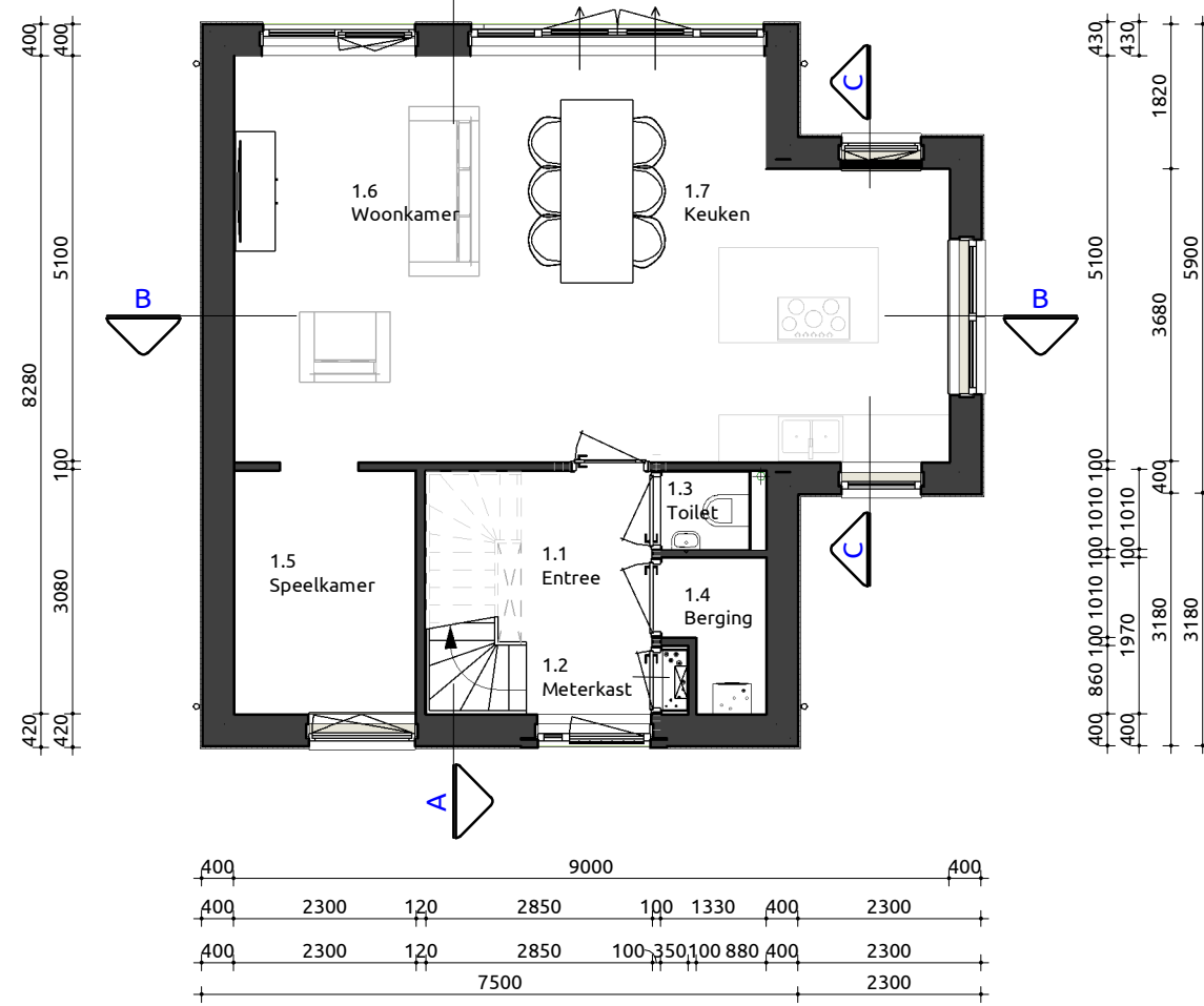
Begane grond 1:100
