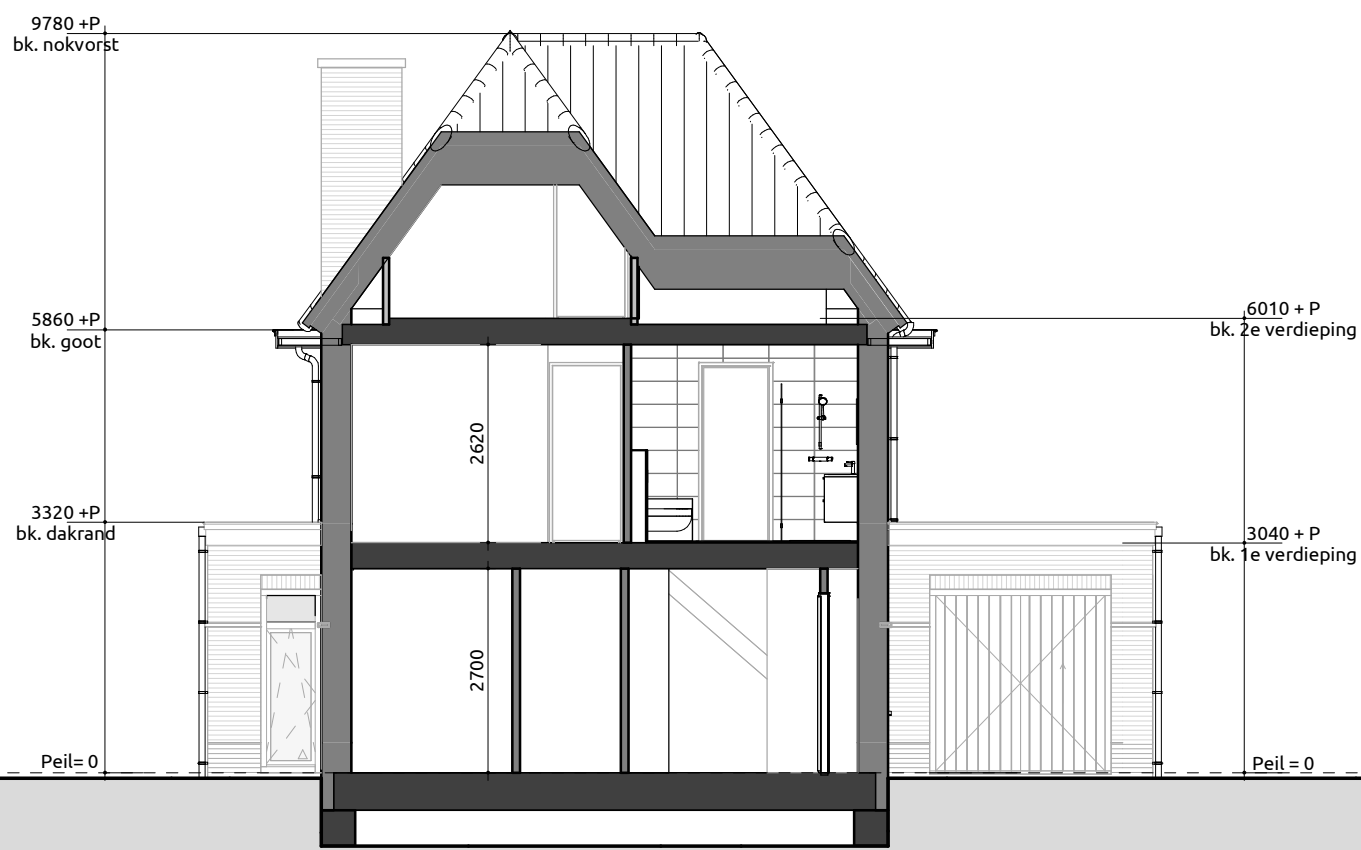
Doorsnede A-A
