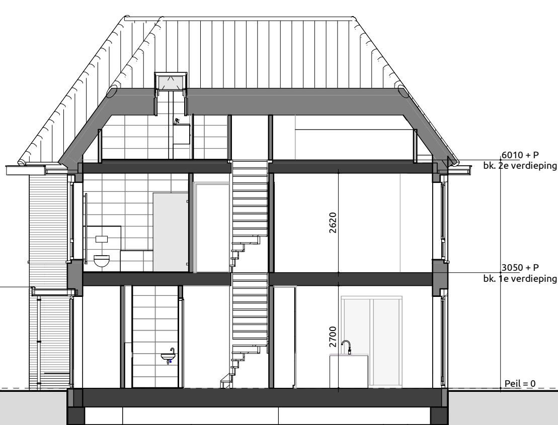
Doorsnede B-B
