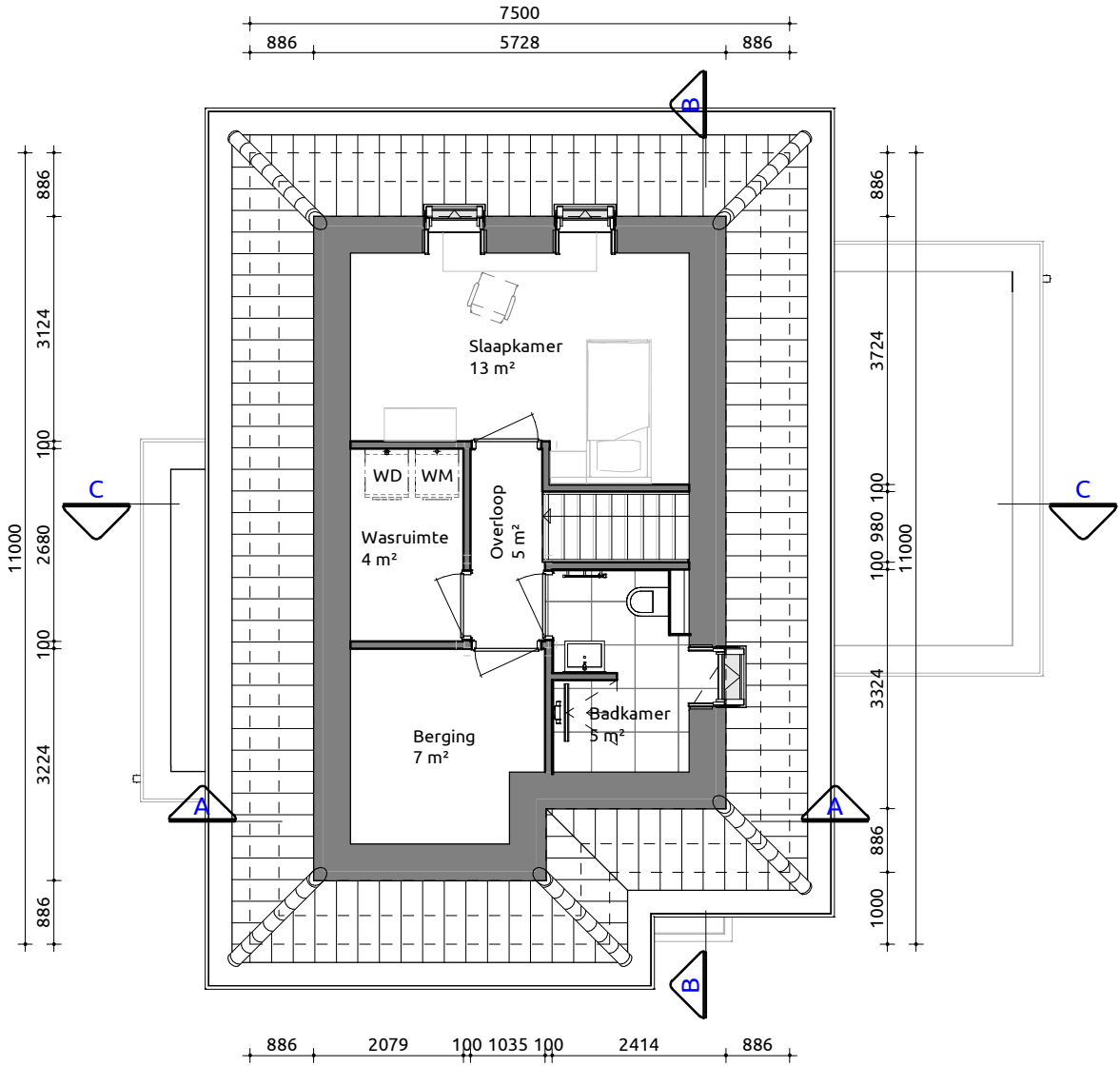
Tweede verdieping
