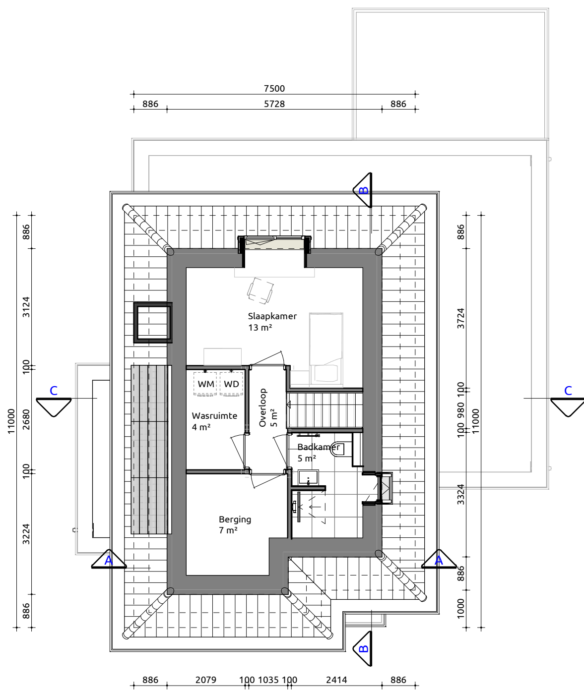
Tweede verdieping
