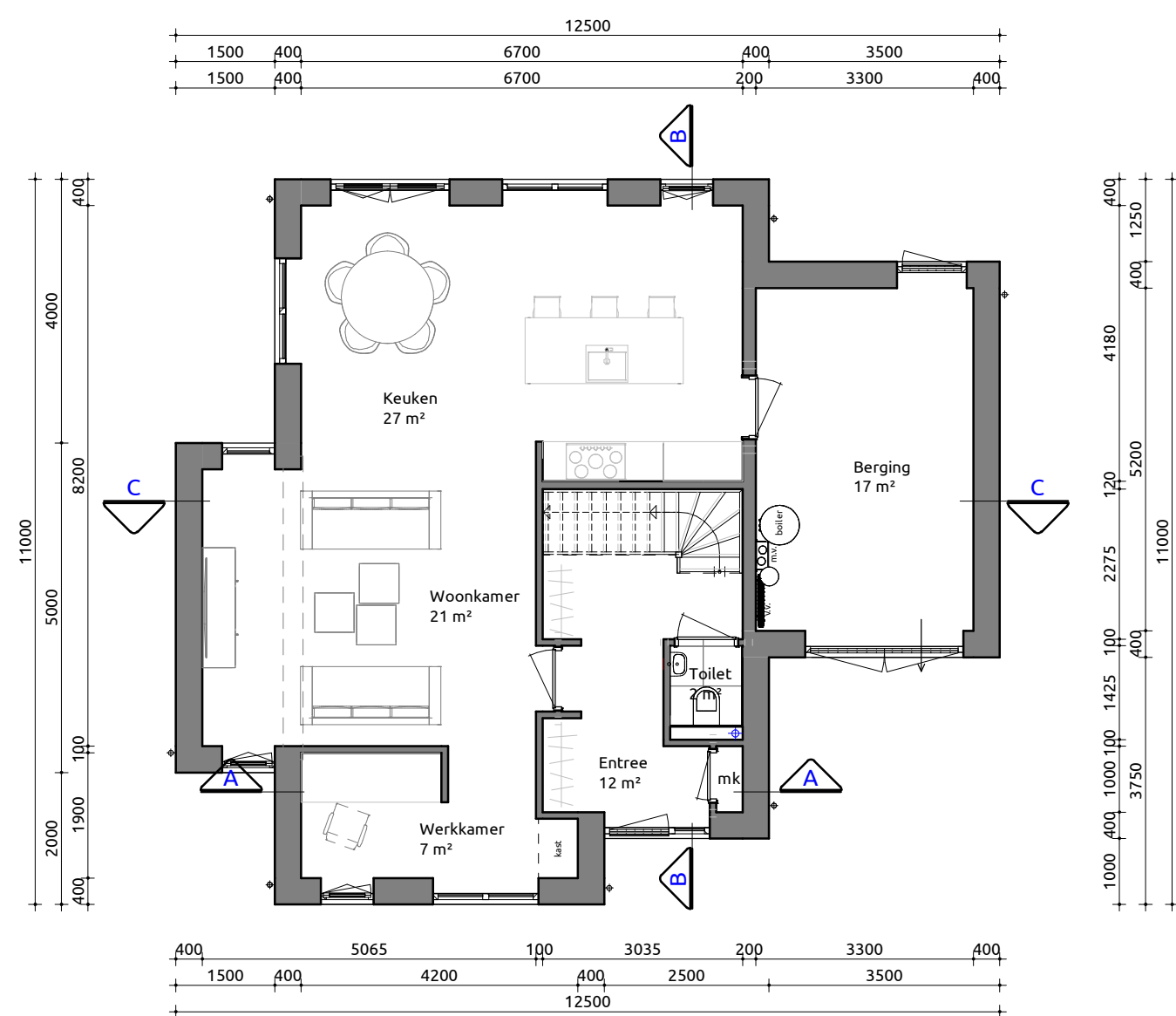
Begane grond
