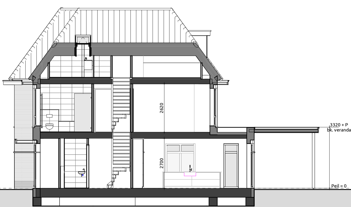
Doorsnede B-B
