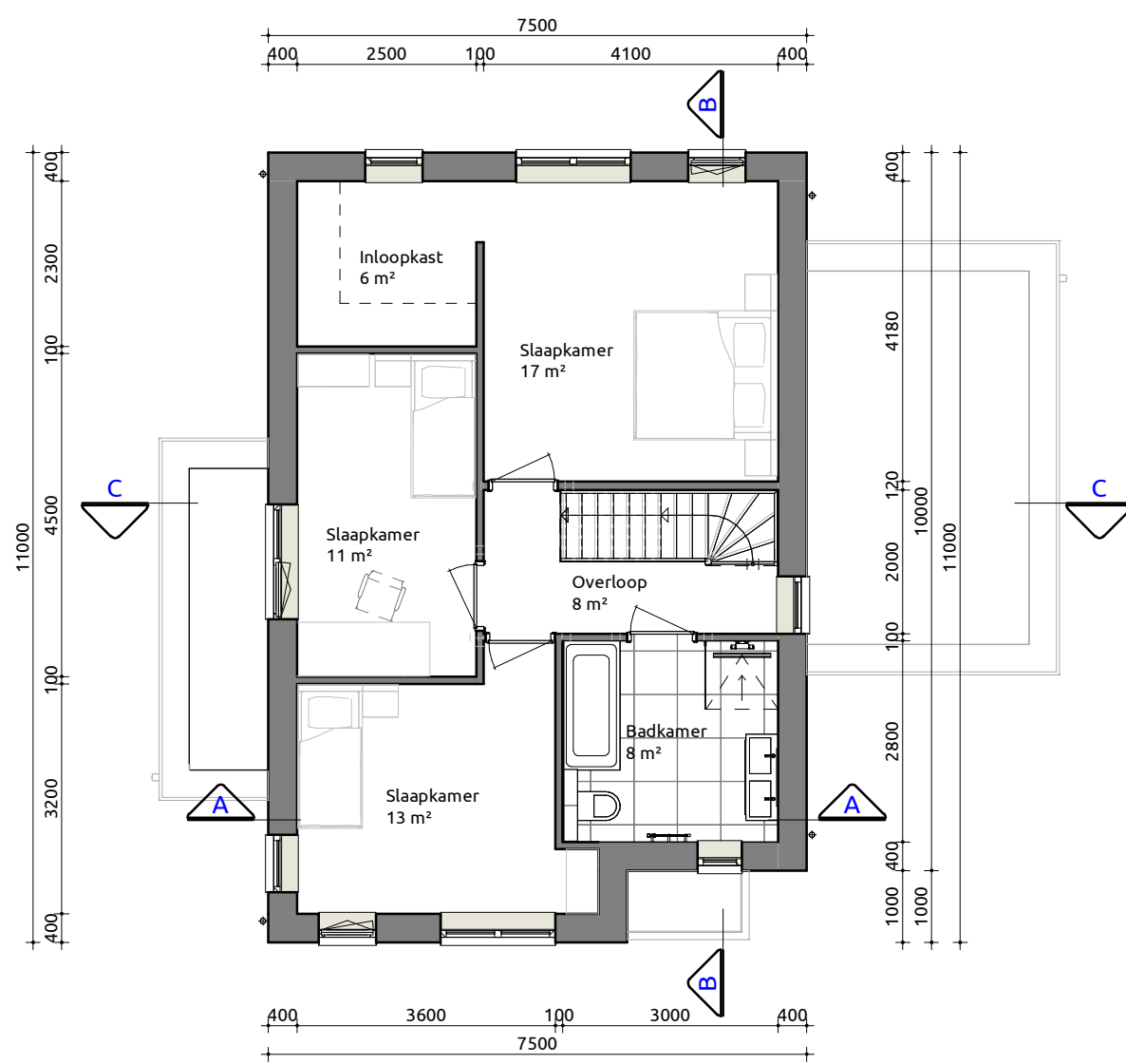
Eerste verdieping
