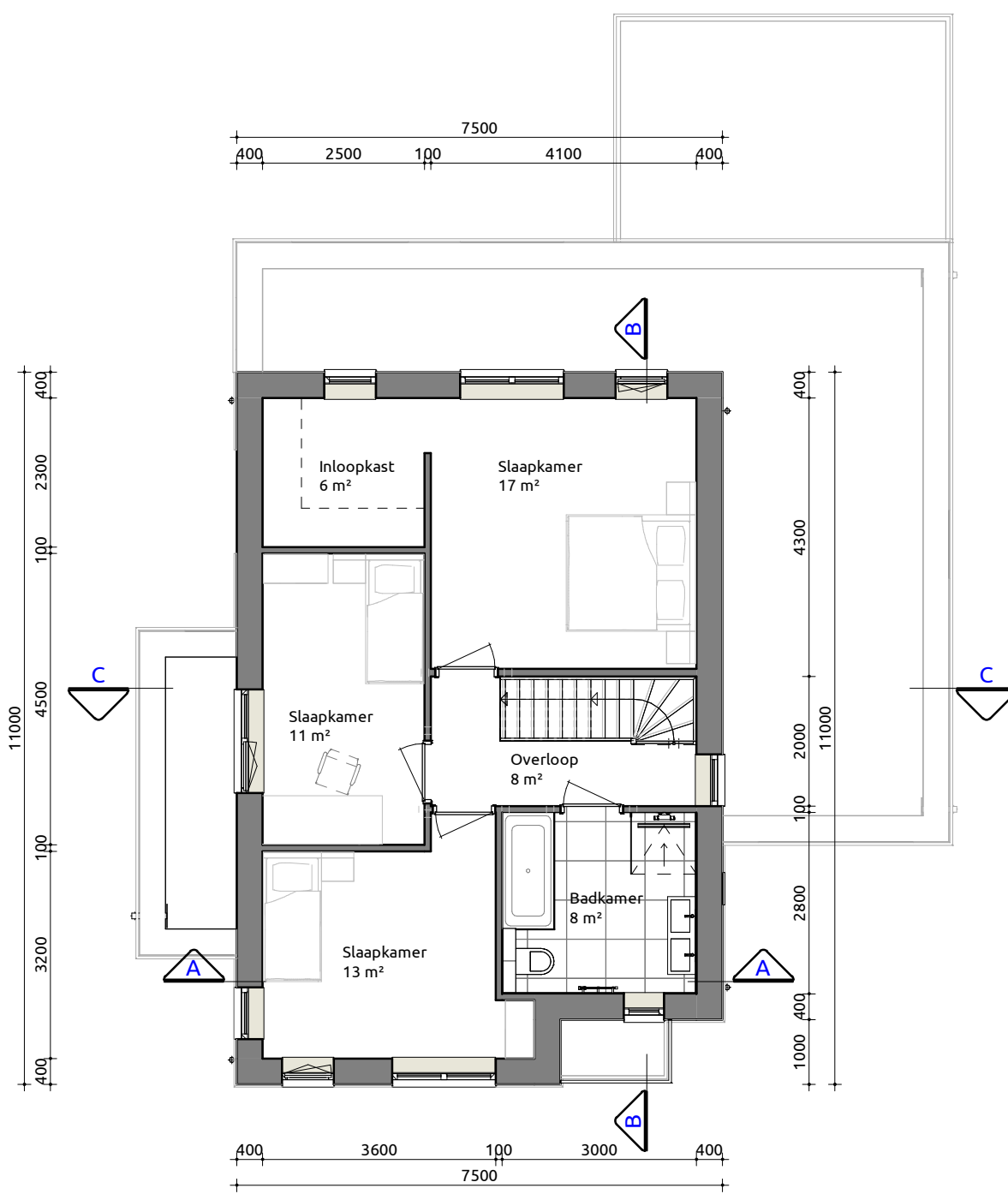
Eerste verdieping
