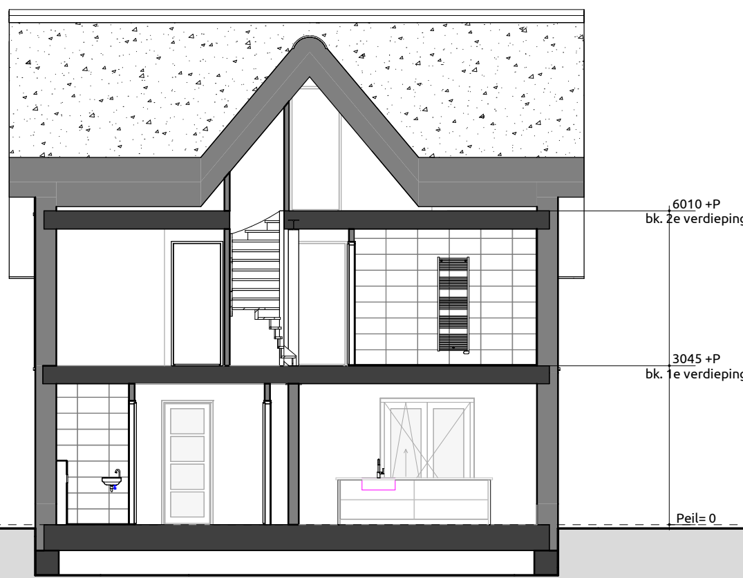
Doorsnede B-B
