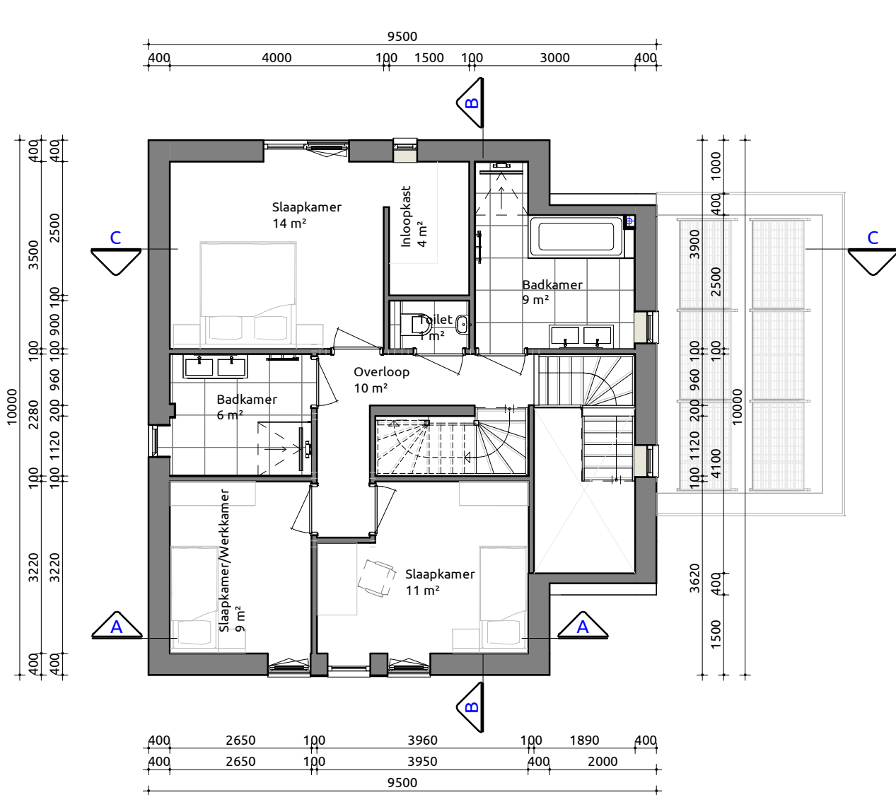
Eerste verdieping
