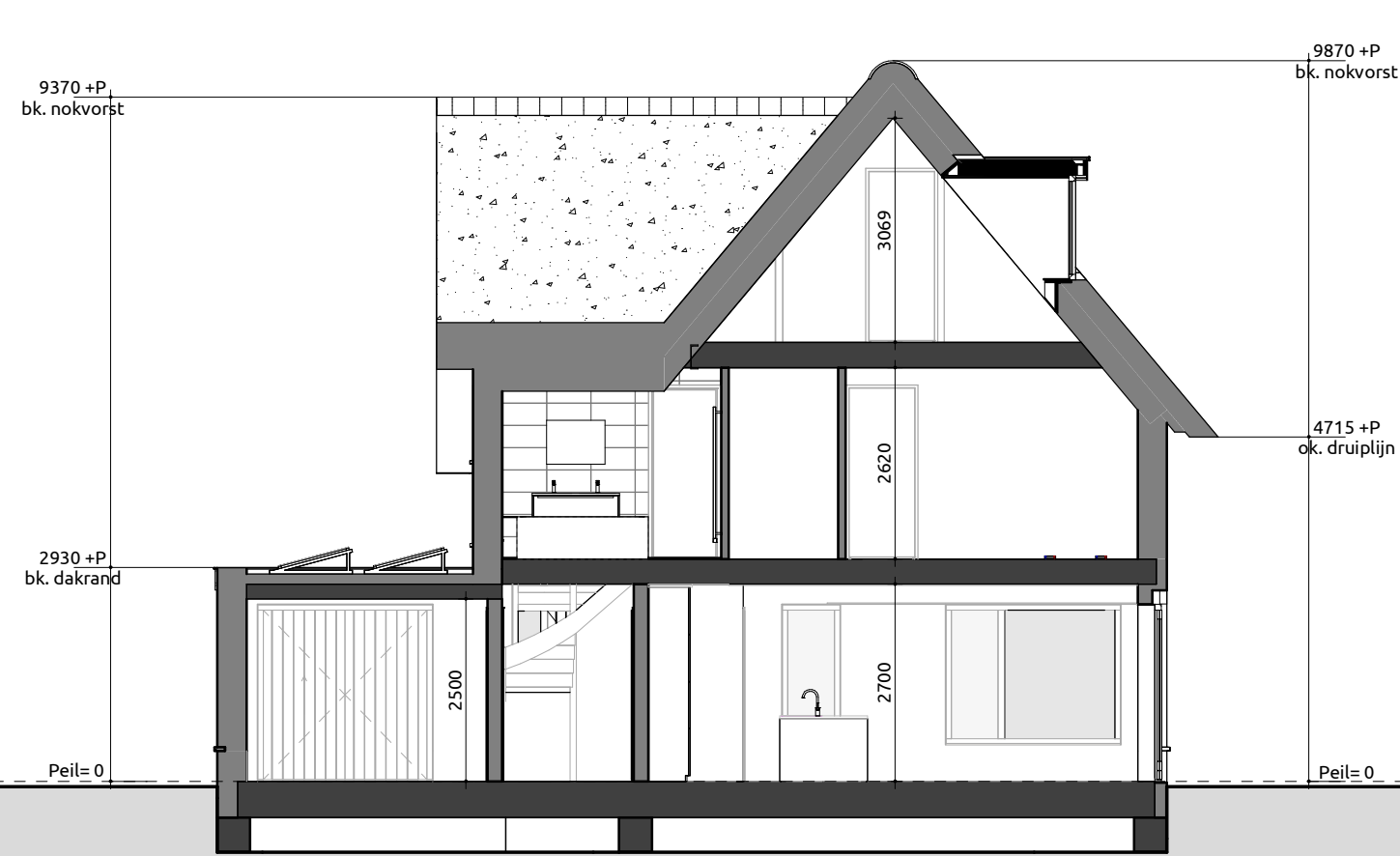
Doorsnede C-C
