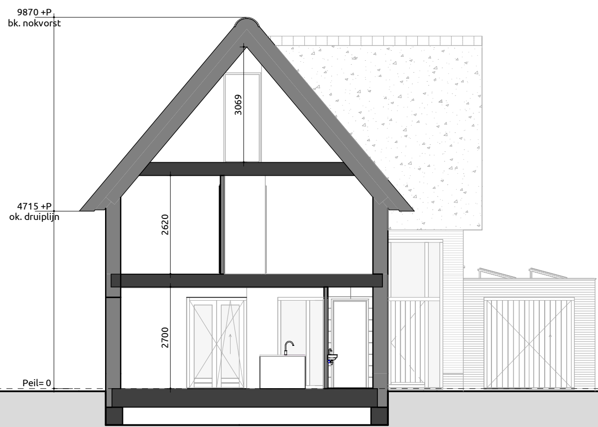
Doorsnede A-A
