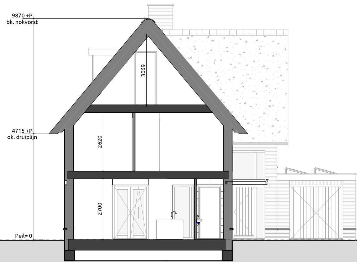
Doorsnede A-A
