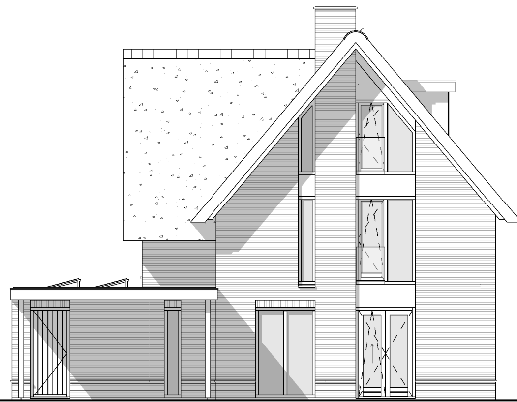
Achtergevel
