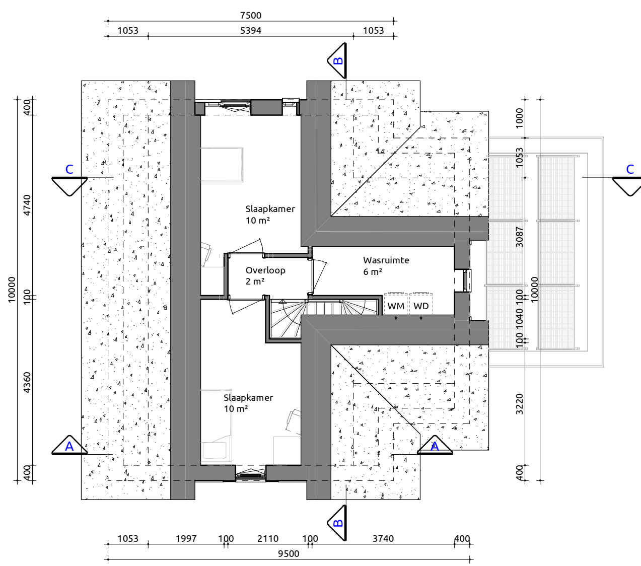
Tweede verdieping
